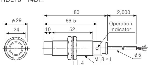
●PRDL18-14D□
